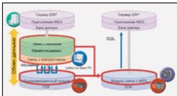
Рис. 3. Устанавливаемый в контроллер модуль связи с MES заменяет собой ненадежный шлюз на базе компьютера с программным обеспечением сторонних производителей
